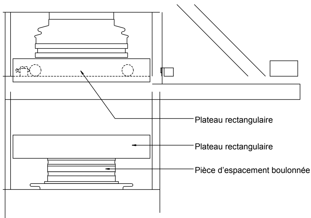
Figure 7.3. Configurer pour tester les blocs nécessitant moins que l'espace vertical maximal
