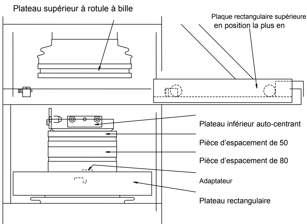
Figure 7.4. Mise en route pour essais sur des cubes de 150 mm
